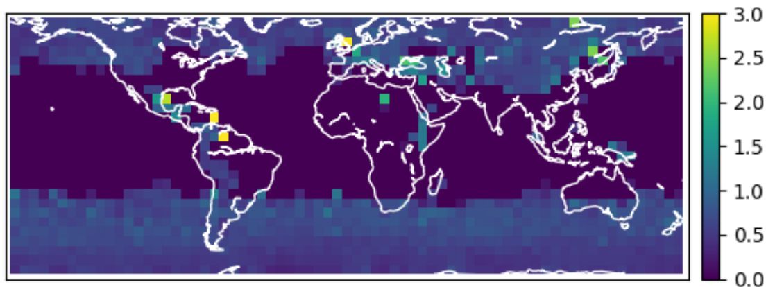
readDPRL3.py 出力例
