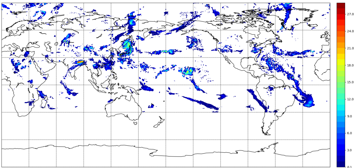
readGSMP_binary.py 出力例
