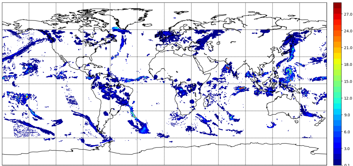
readGSMP_netcdf.py 出力例
