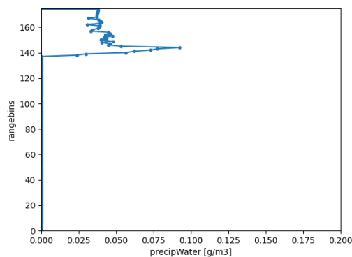
readDPRL2_2.py 出力例
