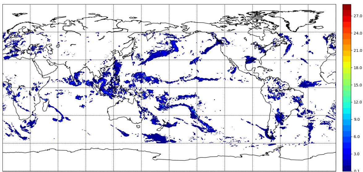
readGSMaP_binary.py 出力例
