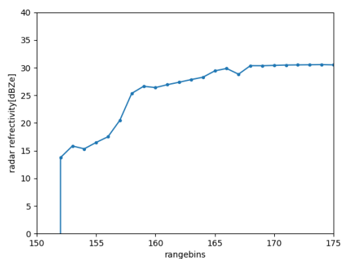
readDPRL2_2.py 出力例
