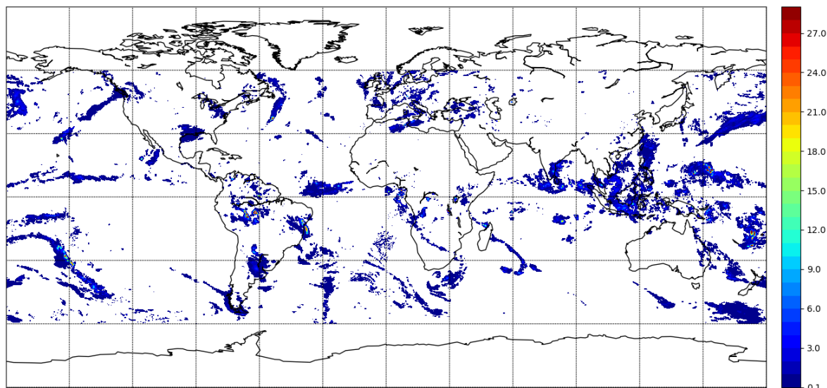
readGSMaP_netcdf.py 出力例
