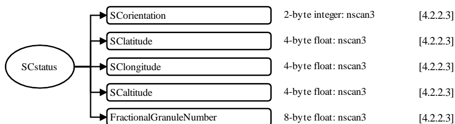
図 4.1-10 1CSSMISのデータフォーマット構造, S3, SCstatus
