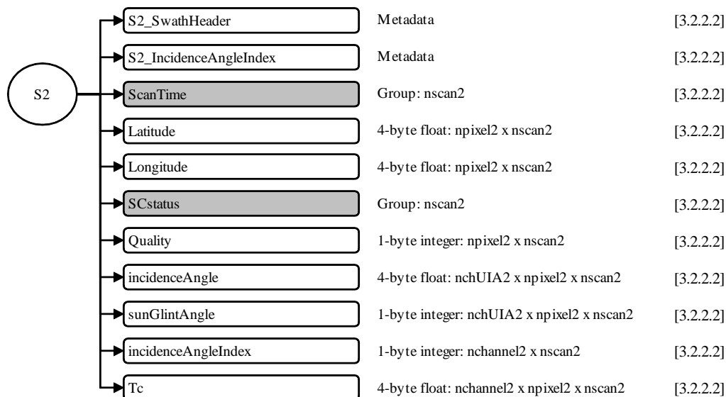
図 3.1-5 1CAMSR2のデータフォーマット構造, S2
