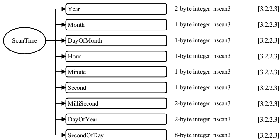
図 3.1-9 1CAMSR2のデータフォーマット構造, S3, ScanTime
