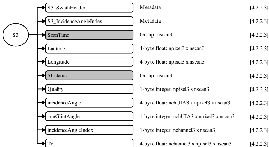
図 4.1-8 1CSSMISのデータフォーマット構造, S3
