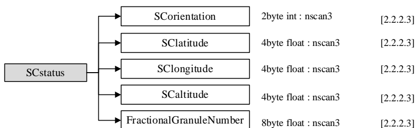
図 2.1-10 1CTMIのデータフォーマット構造, S3,SCstatus
