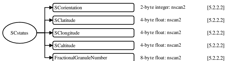
図 5.1-7 1CATMSのデータフォーマット構造, S2,SCstatus
