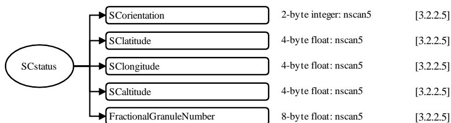
図 3.1-16 1CAMSR2のデータフォーマット構造, S5, SCstatus
