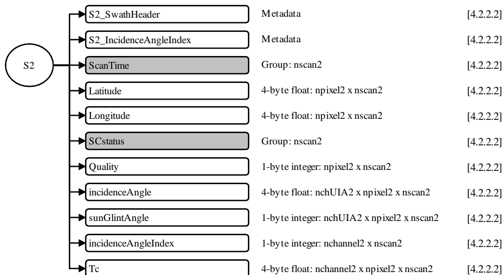
図 4.1-5 1CSSMISのデータフォーマット構造, S2
