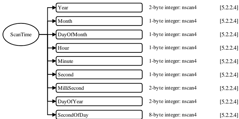
図 5.1-12 1CATMSのデータフォーマット構造, S4, ScanTime
