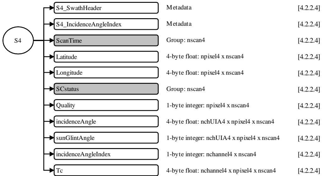
図 4.1-11 1CSSMISのデータフォーマット構造, S4
