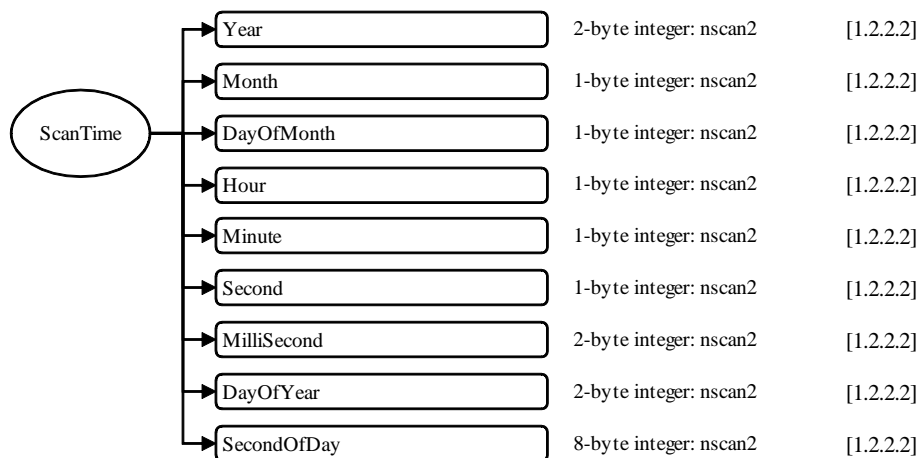
図 1.1-6 ICGMIのデータフォーマット構造, S2, ScanTime
