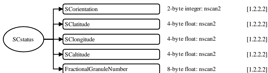
図 1.1-7 ICGMIのデータフォーマット構造, S2, SCstatus
