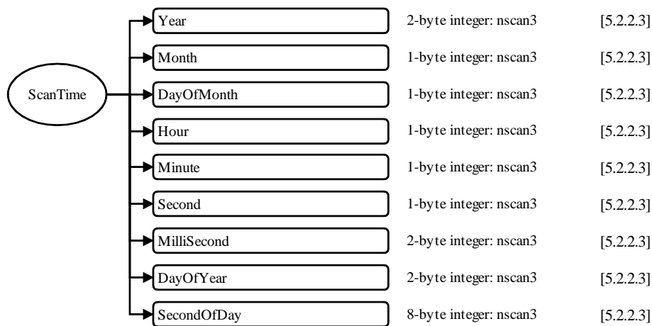
図 5.1-9 1CATMSのデータフォーマット構造, S3,ScanTime
