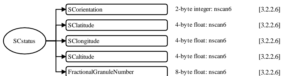
図 3.1-19 1CAMSR2のデータフォーマット構造, S6, SCstatus
