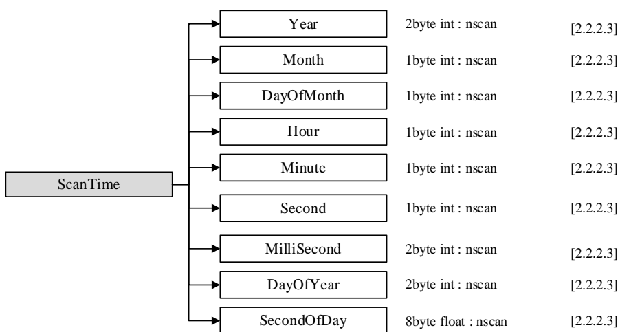
図 2.1-9 1CTMIのデータフォーマット構造, S3,ScanTime
