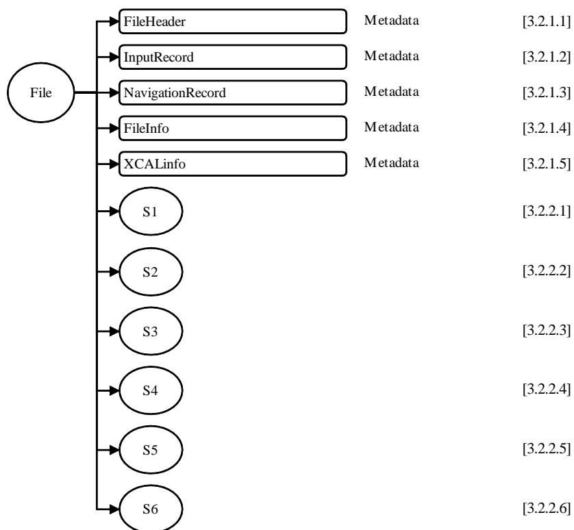
図 3.1-1 1CAMSR2のデータフォーマット構造 - Common Calibrated Brightness Temperature
