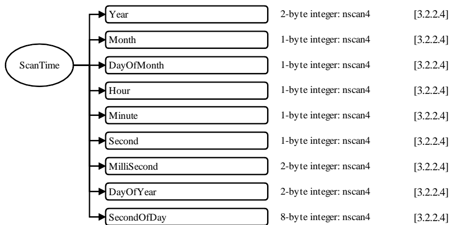
図 3.1-12 1CAMSR2のデータフォーマット構造, S4, ScanTime
