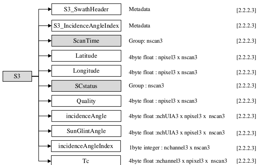
図 2.1-8 1CTMIのデータフォーマット構造, S3
