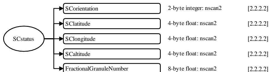
図 2.1-7 1CTMIのデータフォーマット構造, S2, SCstatus
