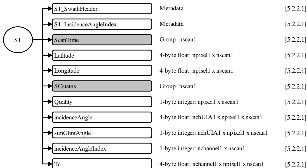
図 5.1-2 1CATMSのデータフォーマット構造, S1
