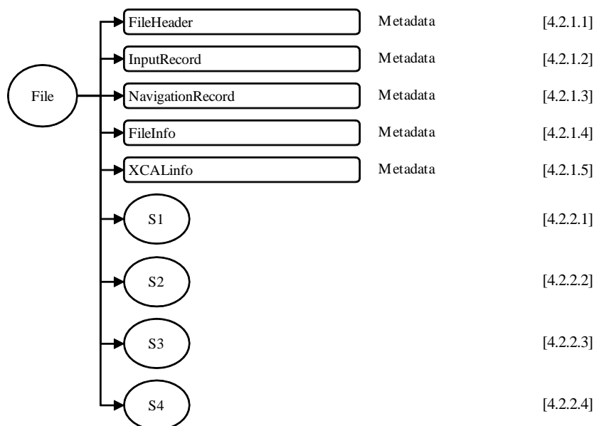
図 4.1-1 1CSSMISのデータフォーマット構造 - Common Calibrated Brightness Temperature
