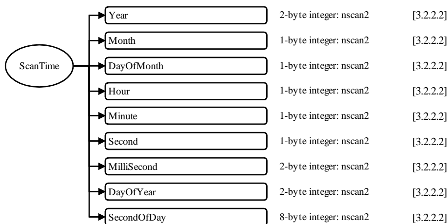
図 3.1-6 1CAMSR2のデータフォーマット構造, S2, ScanTime
