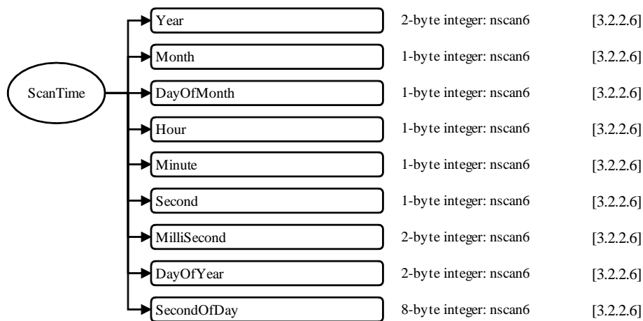
図 3.1-18 1CAMSR2のデータフォーマット構造, S6, ScanTime
