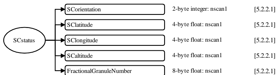
図 5.1-4 1CATMSのデータフォーマット構造, S1, SCstatus
