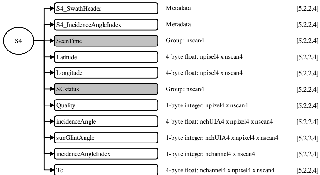
図 5.1-11 1CATMSのデータフォーマット構造, S4
