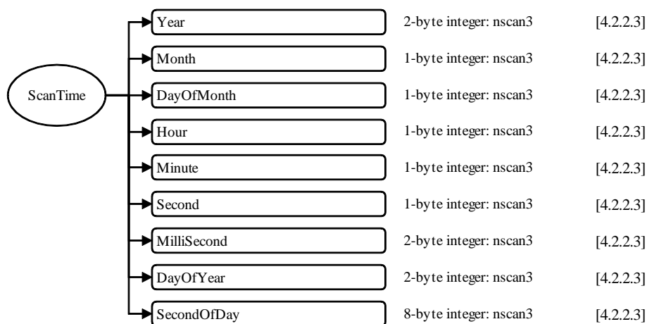
図 4.1-9 1CSSMISのデータフォーマット構造, S3, ScanTime
