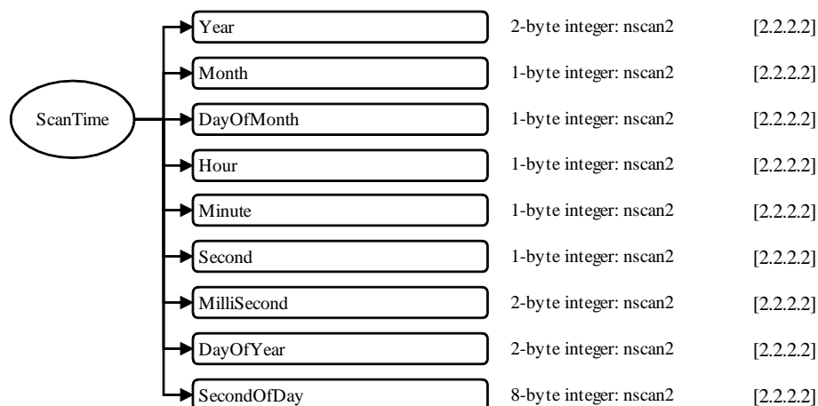
図 2.1-6 1CTMIのデータフォーマット構造, S2, ScanTime
