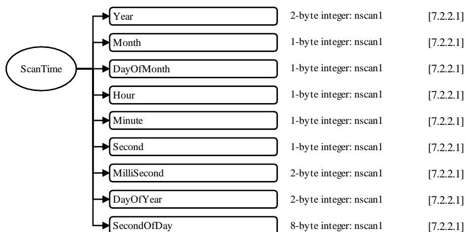
図 7.1-3 1CSAPHIRのデータフォーマット構造, S1, ScanTime
