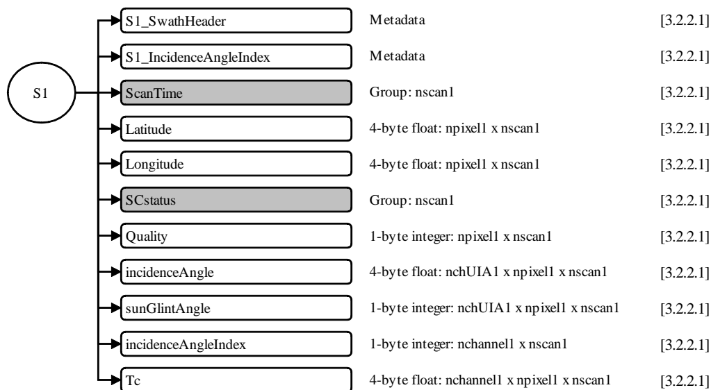
図 3.1-2 1CAMSR2のデータフォーマット構造, S1
