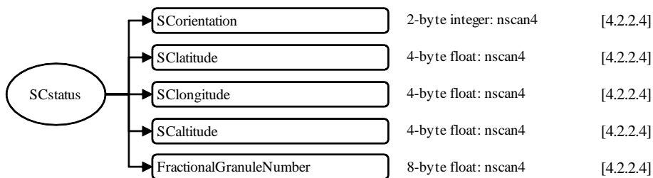
図 4.1-13 1CSSMISのデータフォーマット構造, S4, SCstatus
