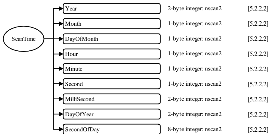
図 5.1-6 1CATMSのデータフォーマット構造, S2,ScanTime
