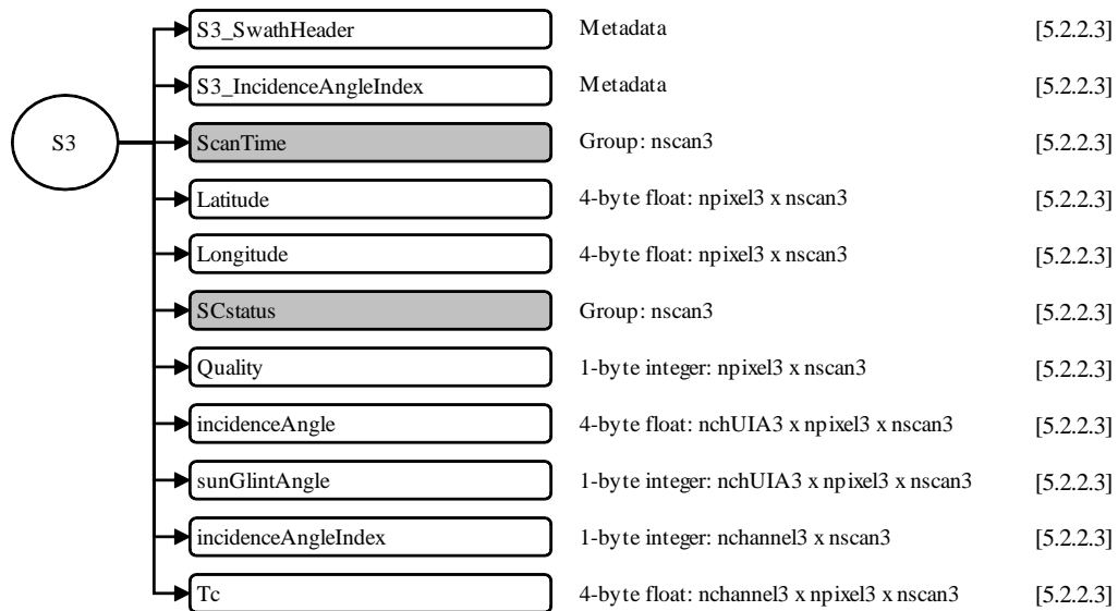
図 5.1-8 1CATMSのデータフォーマット構造, S3
