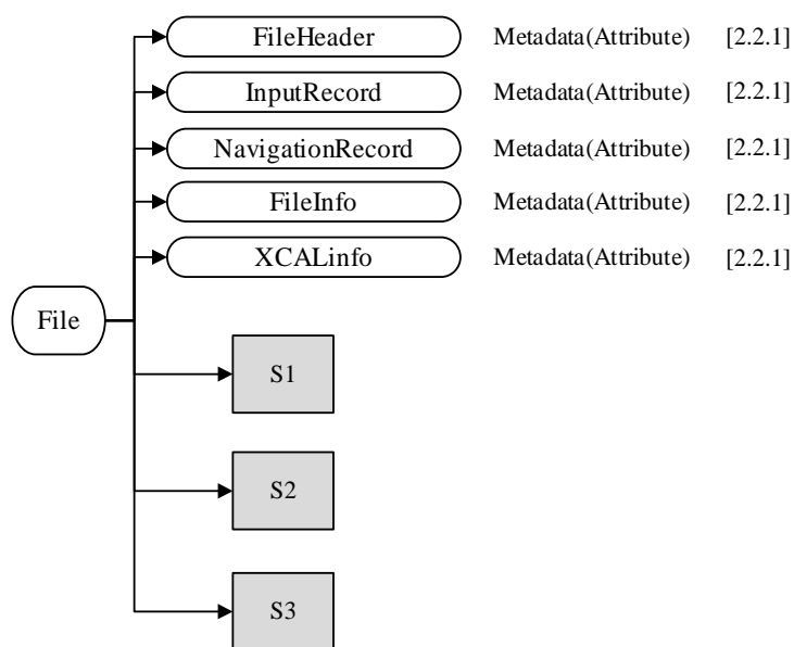
図 2.1-1 ICTMIのデータフォーマット構造 - GPM Common Calibrated Brightness Temperature
