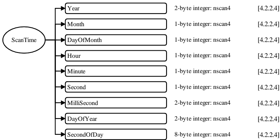
図 4.1-12 1CSSMISのデータフォーマット構造, S4, ScanTime
