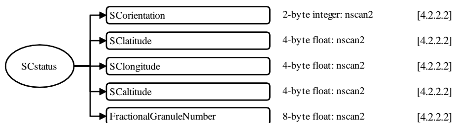
図 4.1-7 1CSSMISのデータフォーマット構造, S2, SCstatus
