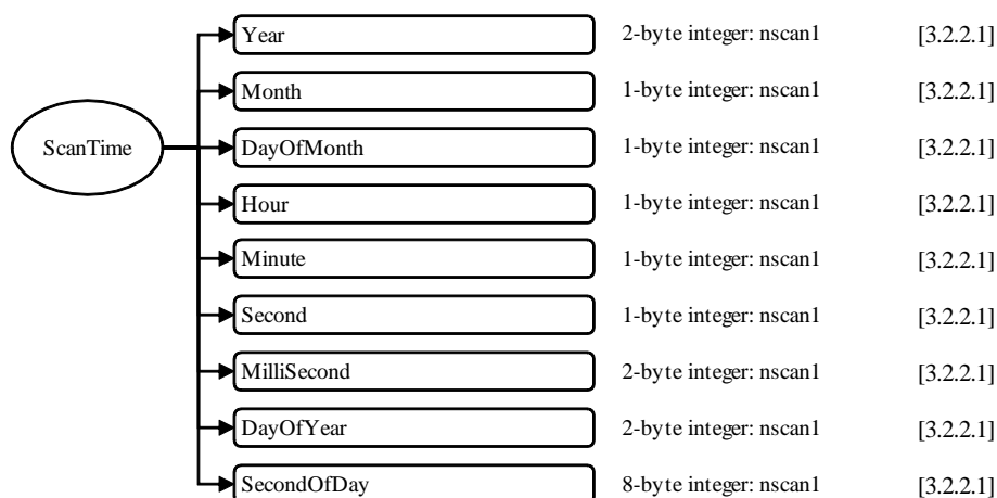
図 3.1-3 1CAMSR2のデータフォーマット構造, S1, ScanTime
