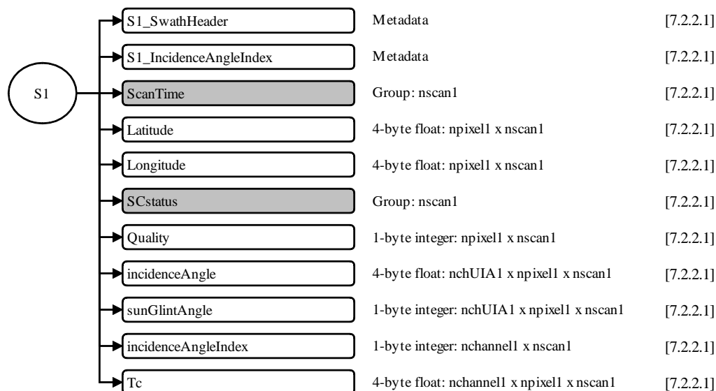
図 7.1-2 1CSAPHIRのデータフォーマット構造, S1
