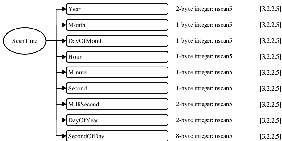
図 3.1-15 1CAMSR2のデータフォーマット構造, S5, ScanTime
