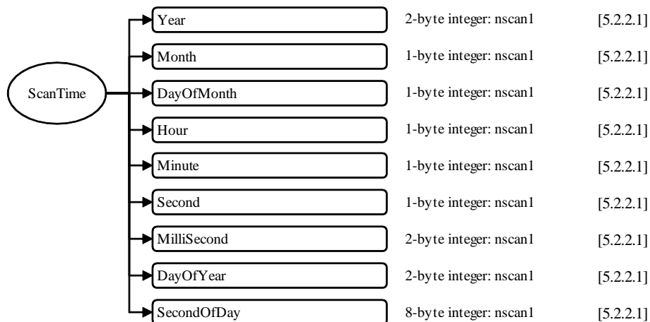
図 5.1-3 1CATMSのデータフォーマット構造, S1,ScanTime
