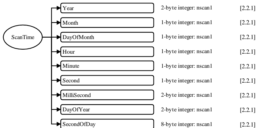
図 2.1-3 1CTMIのデータフォーマット構造, S1,ScanTime
