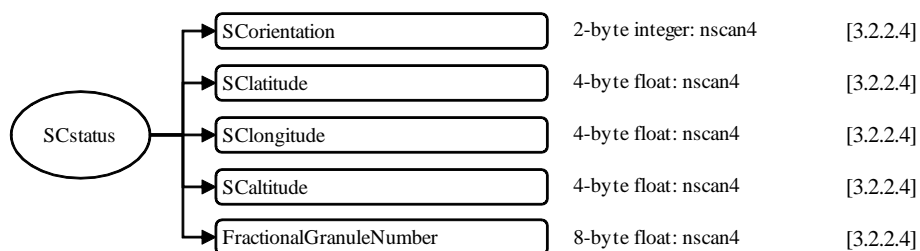
図 3.1-13 1CAMSR2のデータフォーマット構造, S4, SCstatus
