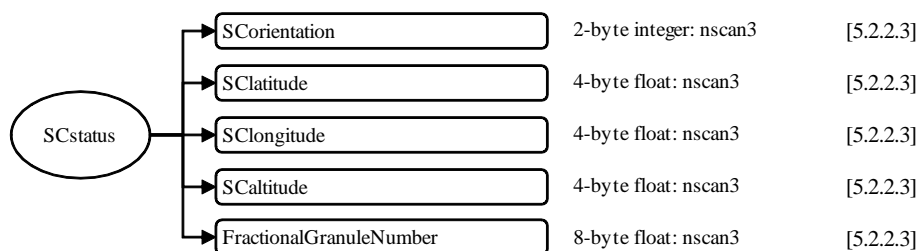
図 5.1-10 1CATMSのデータフォーマット構造, S3,SCstatus
