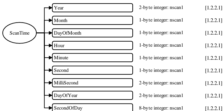
図 1.1-3 ICGMIのデータフォーマット構造, S1, ScanTime
