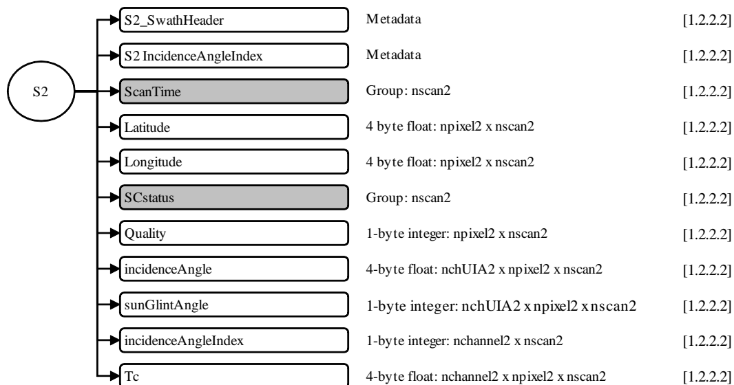
図 1.1-5 ICGMIのデータフォーマット構造, S2
