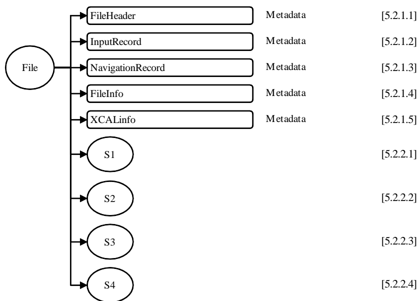
図 5.1-1 1CATMSのデータフォーマット構造 - Common Calibrated Brightness Temperature
