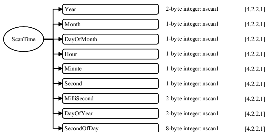
図 4.1-3 1CSSMISのデータフォーマット構造, ScanTime
