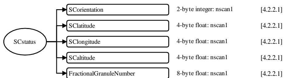
図 4.1-4 1CSSMISのデータフォーマット構造, SCstatus
