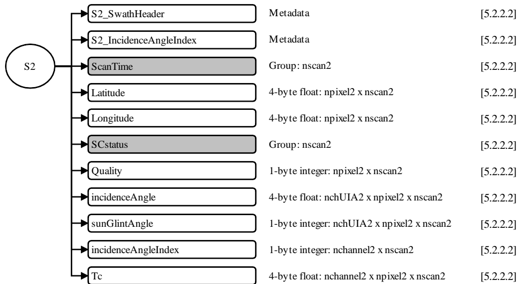
図 5.1-5 1CATMSのデータフォーマット構造, S2
