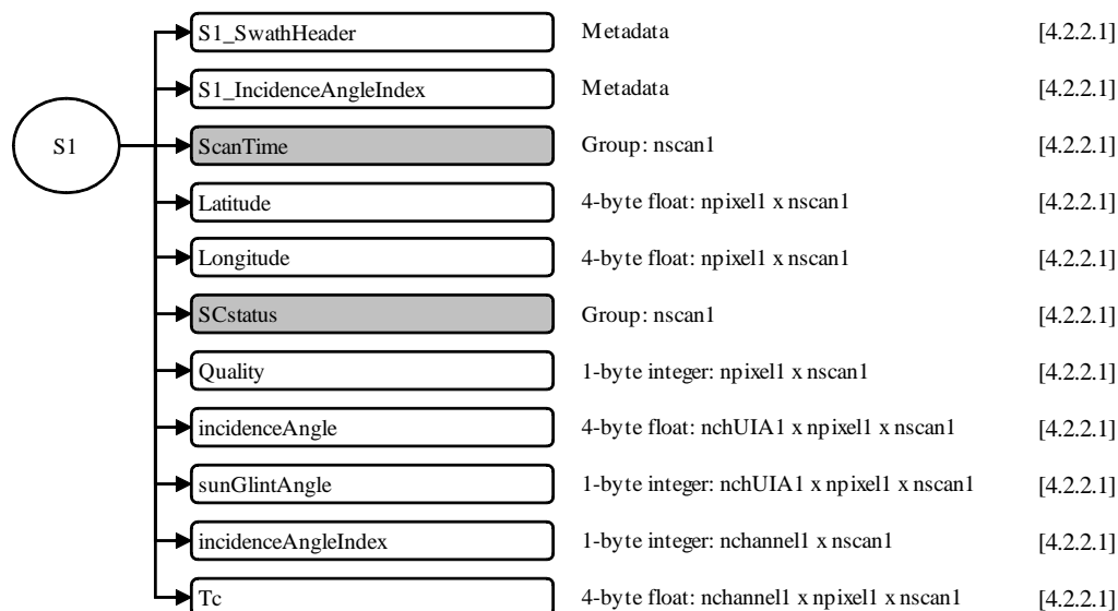
図 4.1-2 1CSSMISのデータフォーマット構造, S1
