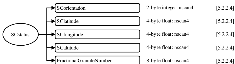
図 5.1-13 1CATMSのデータフォーマット構造, S4, SCstatus
