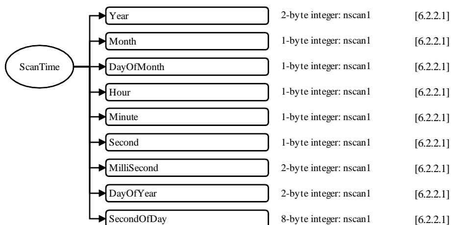
図 6.1-3 1CMHSのデータフォーマット構造, S1, ScanTime
