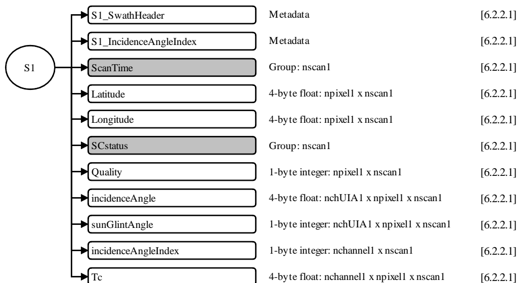
図 6.1-2 1CMHSのデータフォーマット構造, S1
