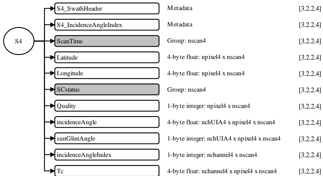
図 3.1-11 1CAMSR2のデータフォーマット構造, S4
