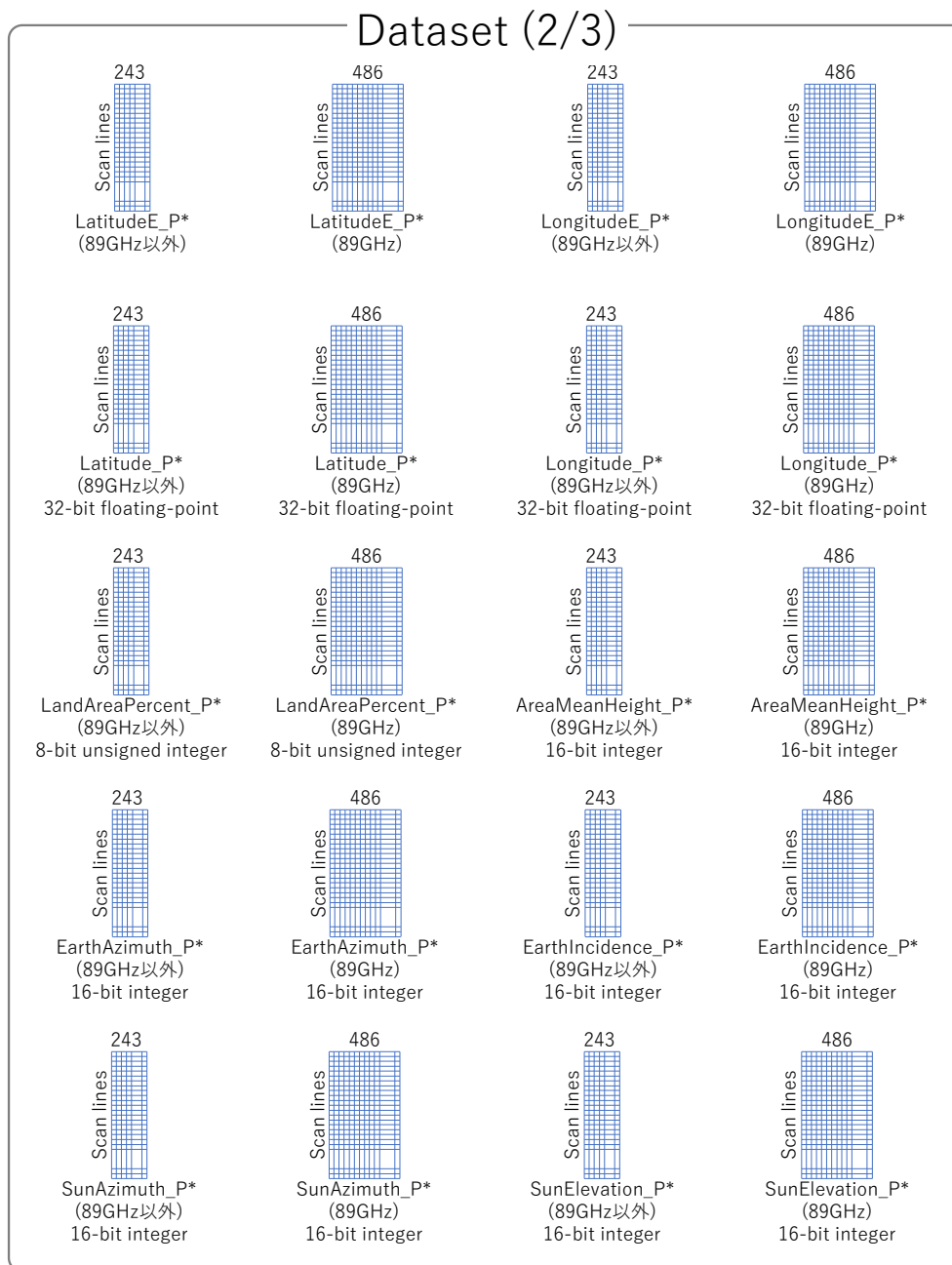
図 3-1 レベル 1 A プロダクトのデータ構成 (2/3)
