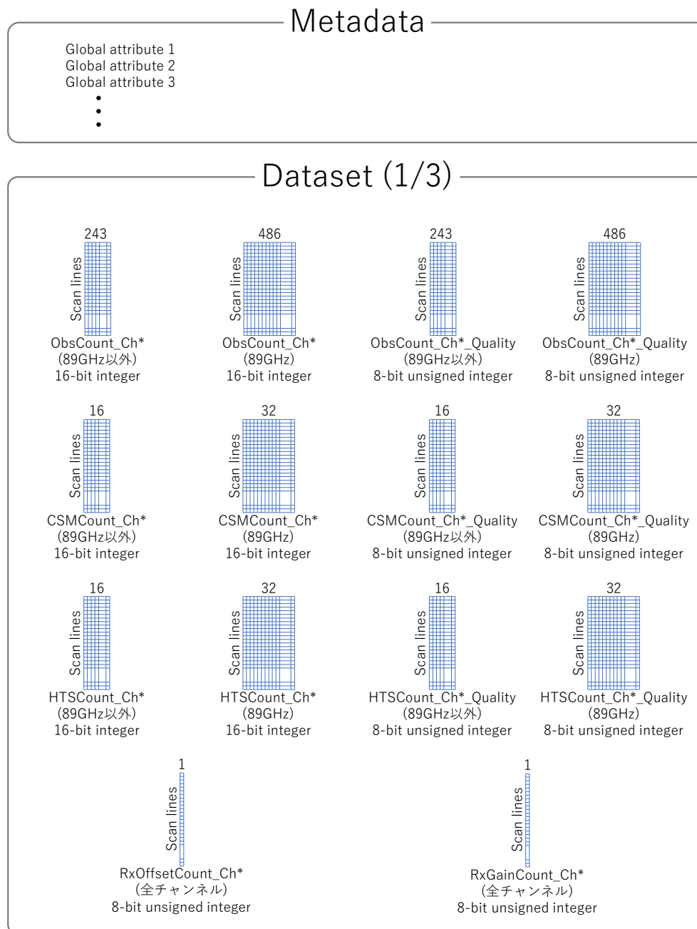
図 3-1 レベル1A プロダクトのデータ構成 (1/3)
