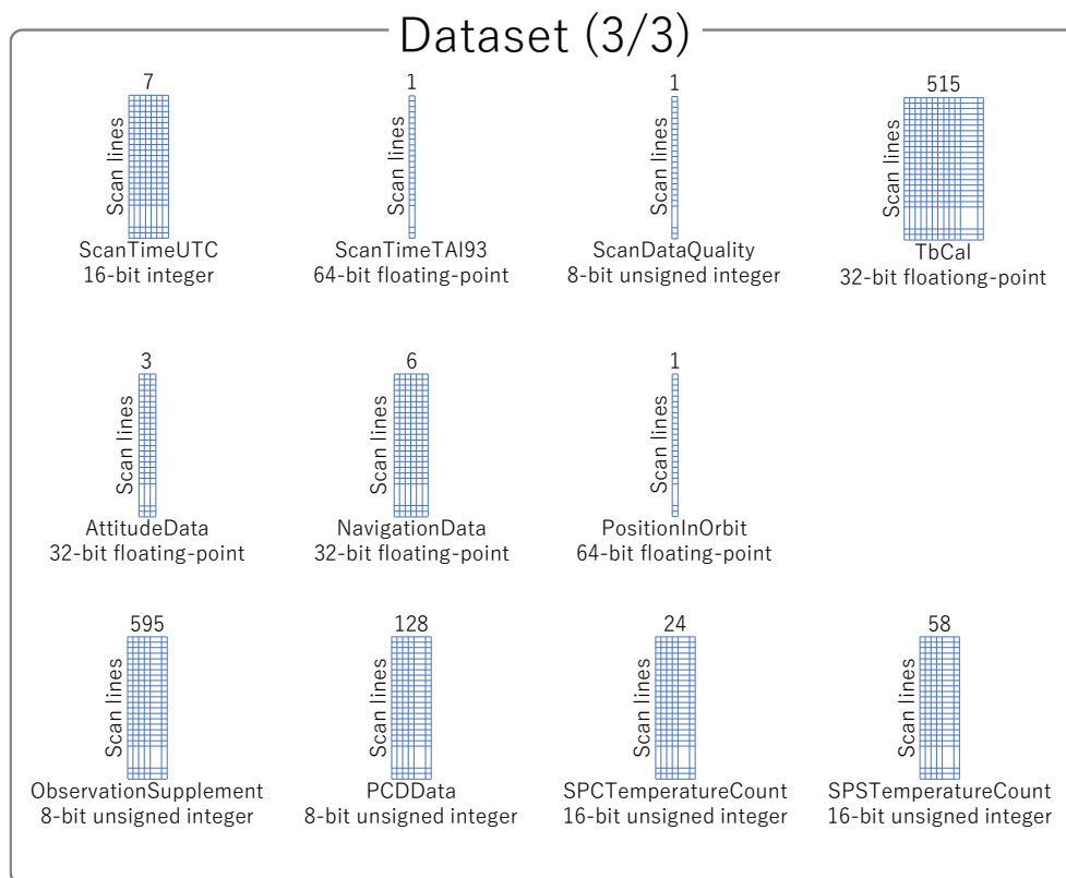
図 3-1 レベル 1 A プロダクトのデータ構成 (3/3)
