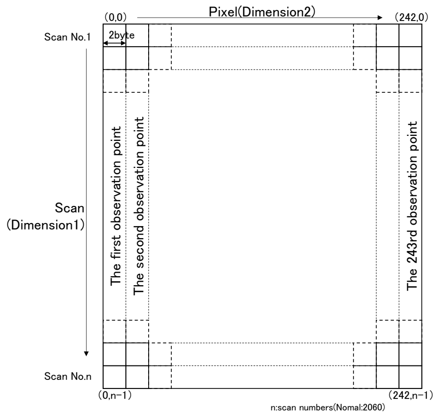
図 3-2 ObsCount(89GHz 以外)の構造
