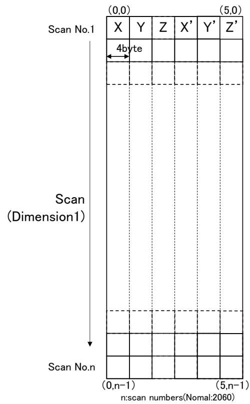
Figure 3-26 NavigationData (Dataset Name : NavigationData)
