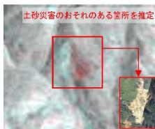
衛星画像を用いた土砂災害判読図
