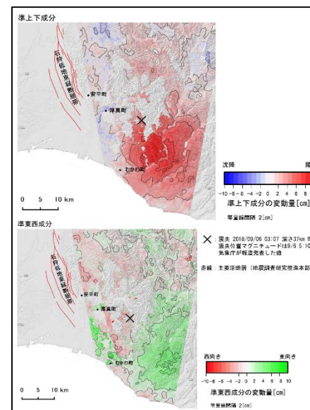
平成30北海道胆振東部地震「だいち2号」による地殻変動分布図(2.5次元解析)(暫定) 平成30年9月11日地震調査研究推進本部地震調査委員会発表資料「平成30年北海道胆振東部地震の評価」より抜粋
