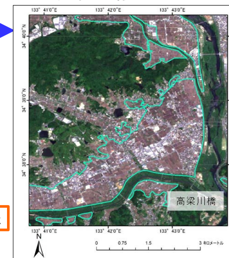
災害域抽出情報の例
