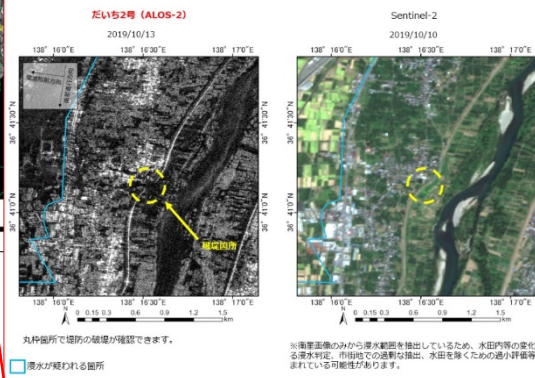
No.2 破堤箇所拡大(長野県長野市、須坂市(千曲川流域))
