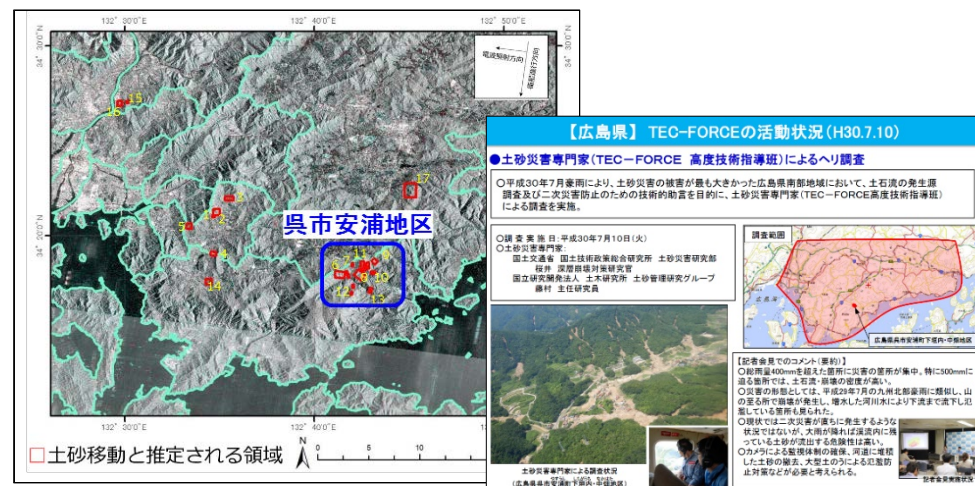
崩壊発生箇所抽出例(広島県呉市周辺)
