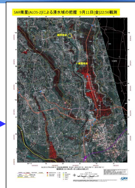
災害速報図の例
