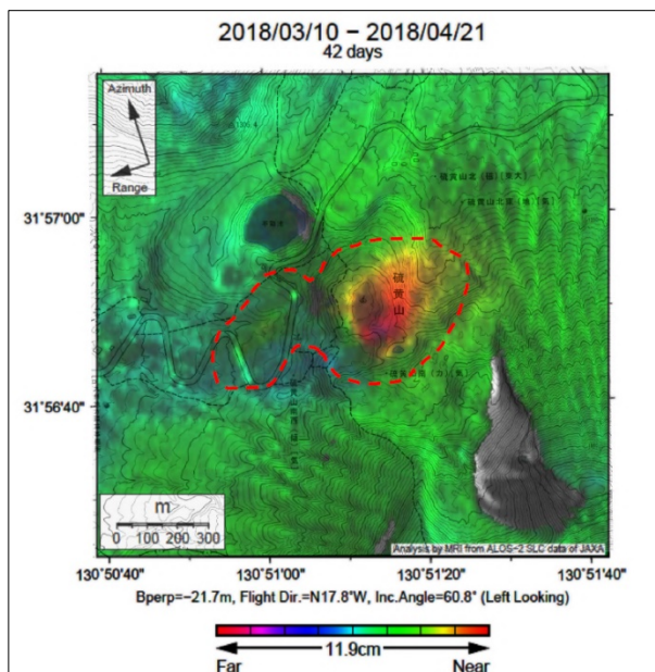
霧島山(えびの高原(硫黄山)周辺) だいち2号干渉SARによる変動
