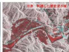
衛星画像を用いた浸水域判読図
