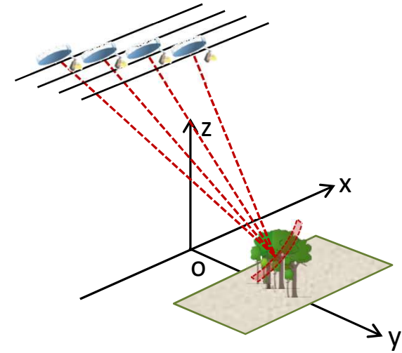
TomoSAR
